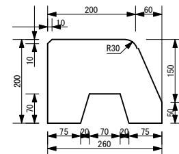
標準縁石
