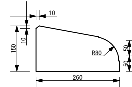
低下縁石
