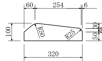
低下縁石
