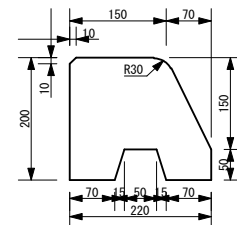
標準縁石
