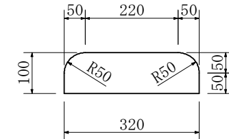
低下縁石
