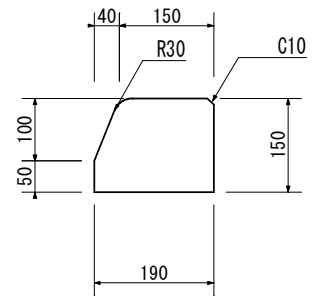
標準縁石
