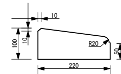
低下縁石
