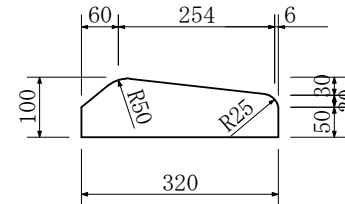
低下縁石
