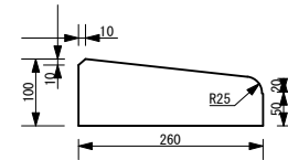
低下縁石
