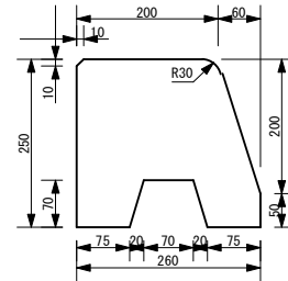
標準縁石
