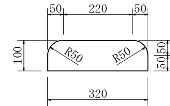
低下縁石
