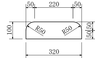
低下縁石
