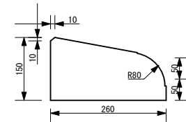
低下縁石
