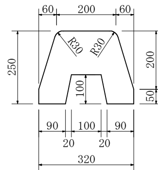
標準縁石
