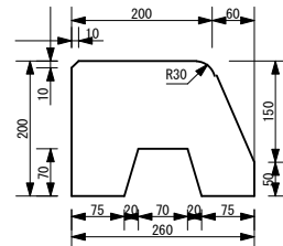
標準縁石
