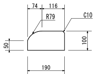
変形B型
