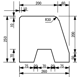
標準縁石
