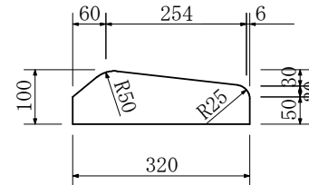
低下縁石
