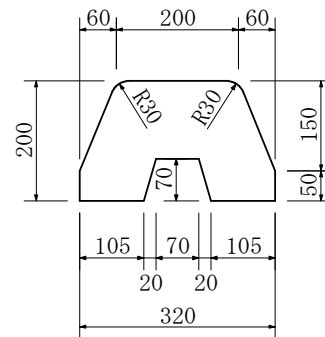
標準縁石
