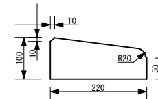
低下縁石
