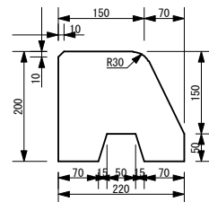
標準縁石
