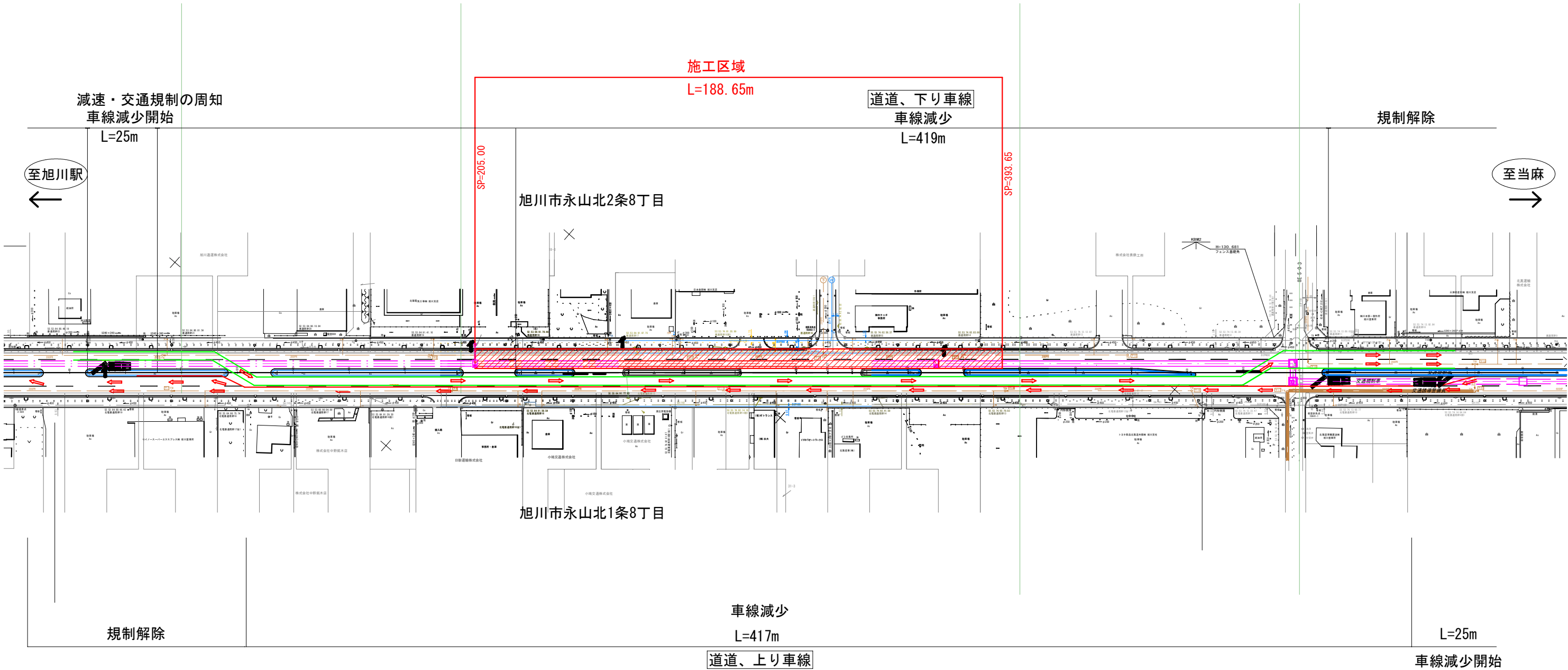
交通規制平面図
