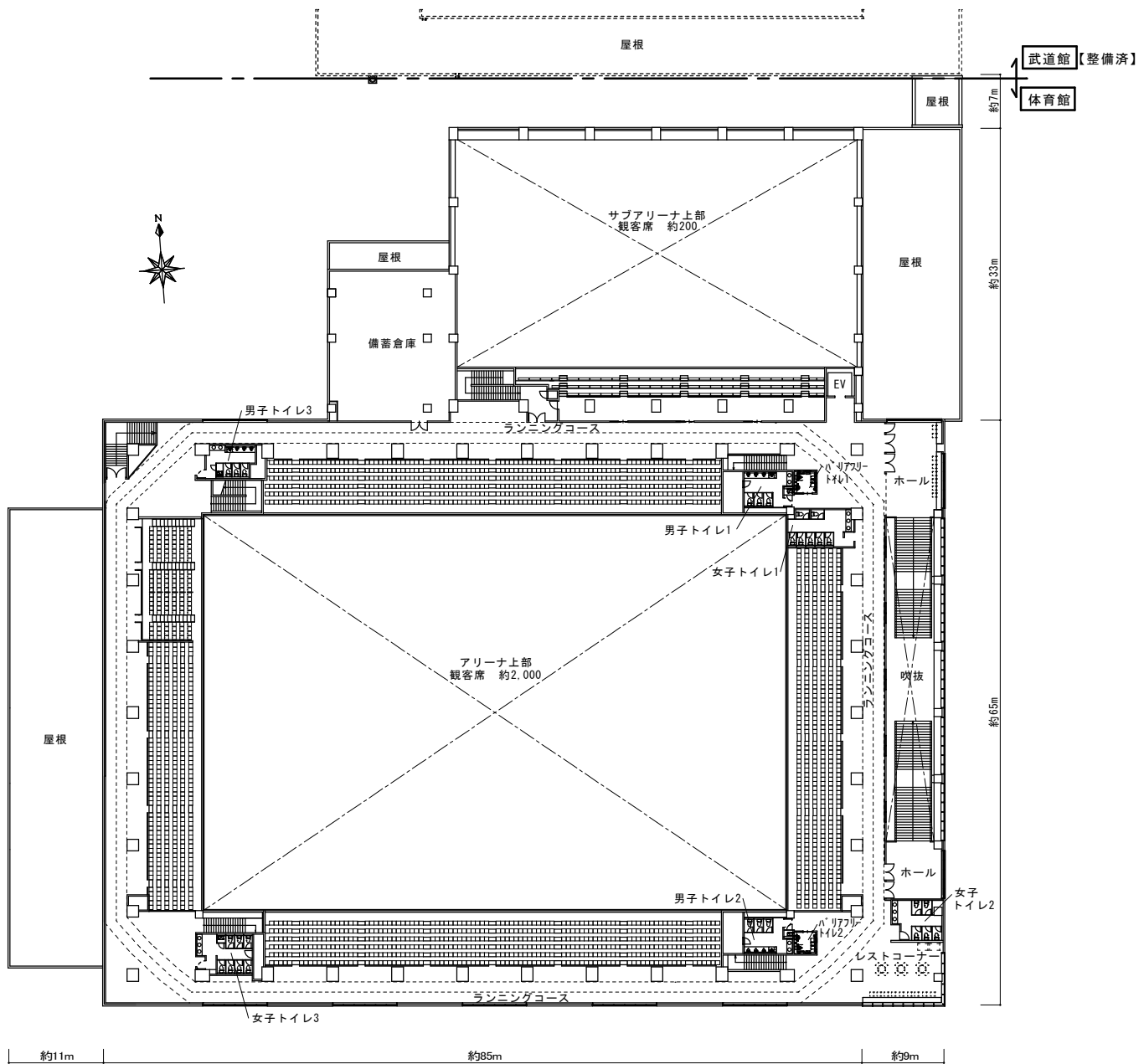
2階平面図 (令和8年4月時点)
