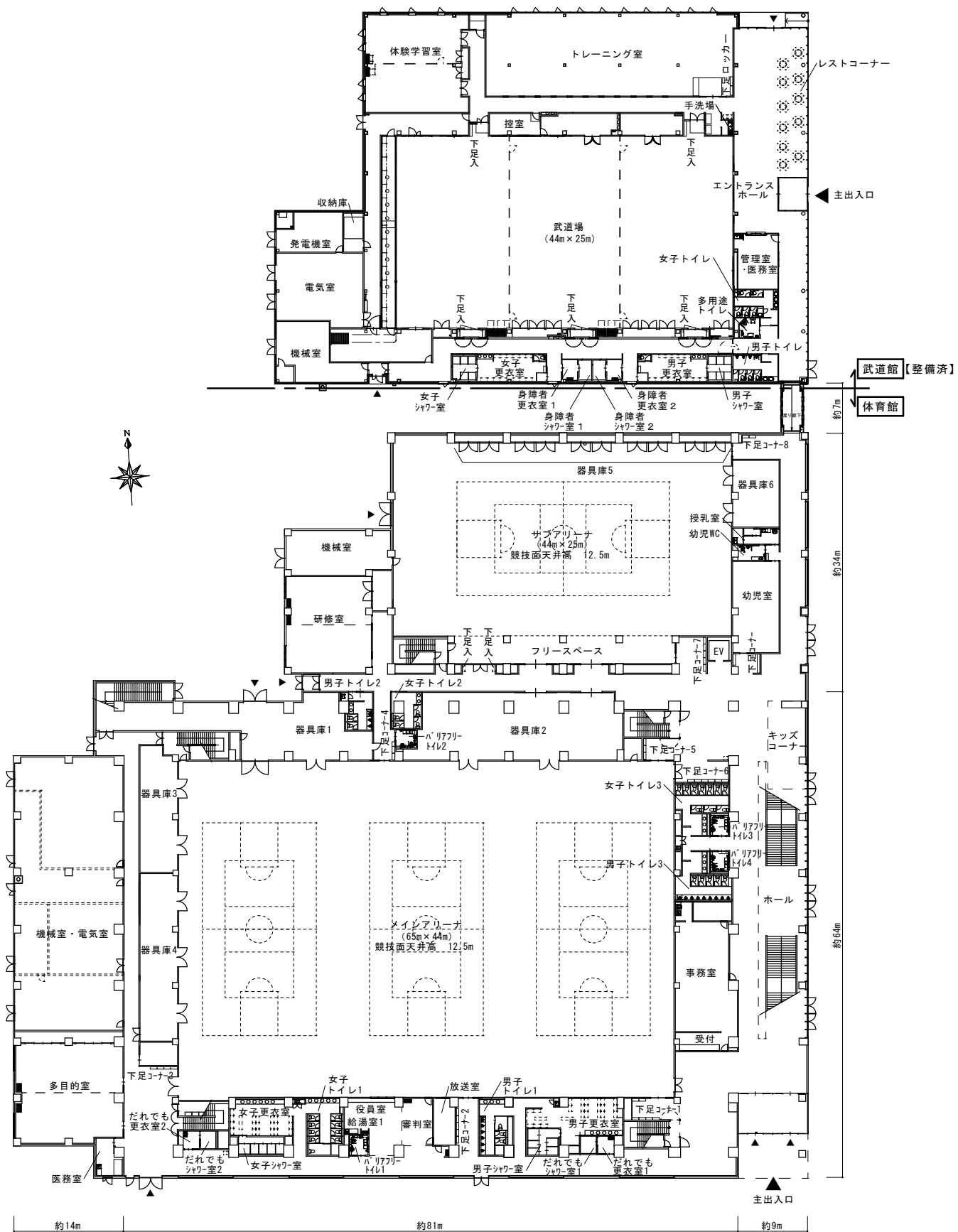
1階平面図 (令和8年4月時点)
