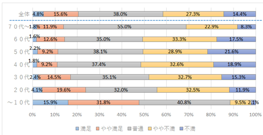
【調査合計】 N=2,258
