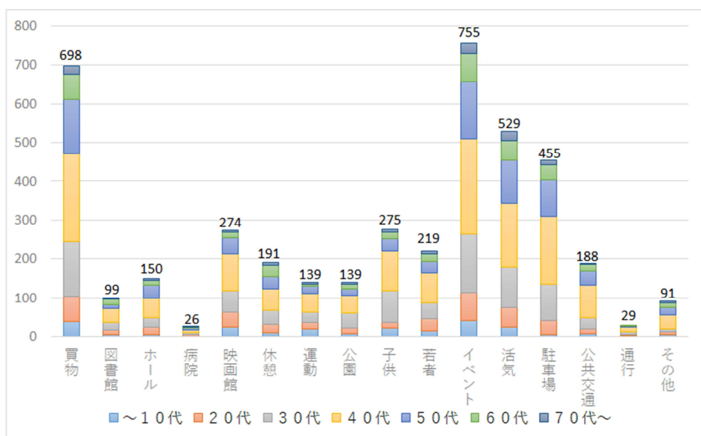
【調査合計】 N=940
