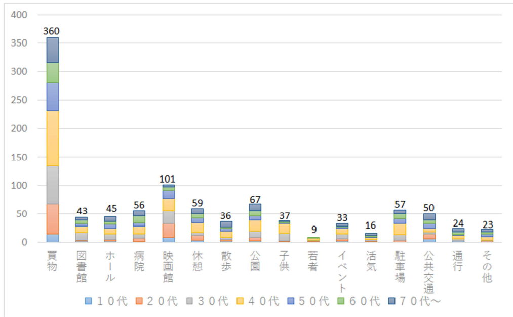
【無作為抽出】N=435
