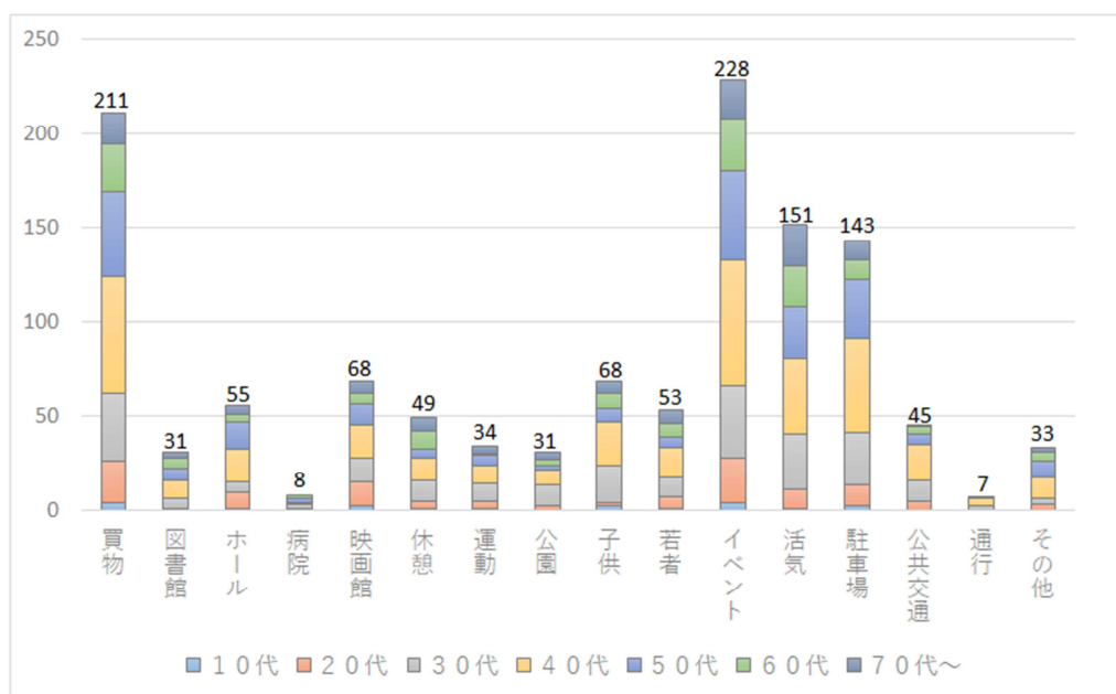
【無作為抽出】 N=283
