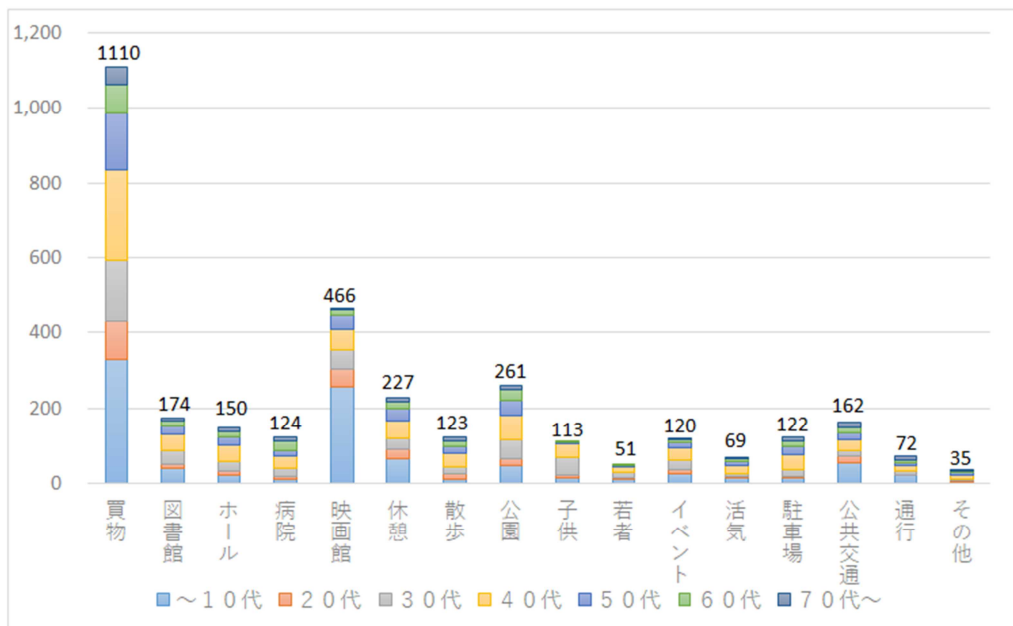
【調査合計】N=1,308
