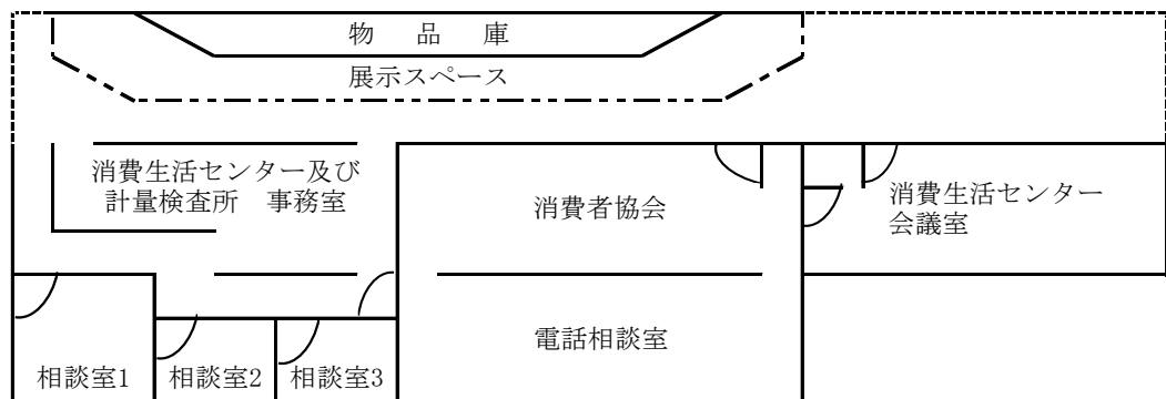
平面図
