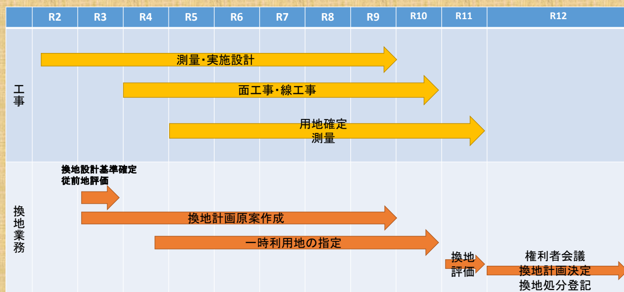
豊台西神楽地区の工事・換地業務スケジュール
