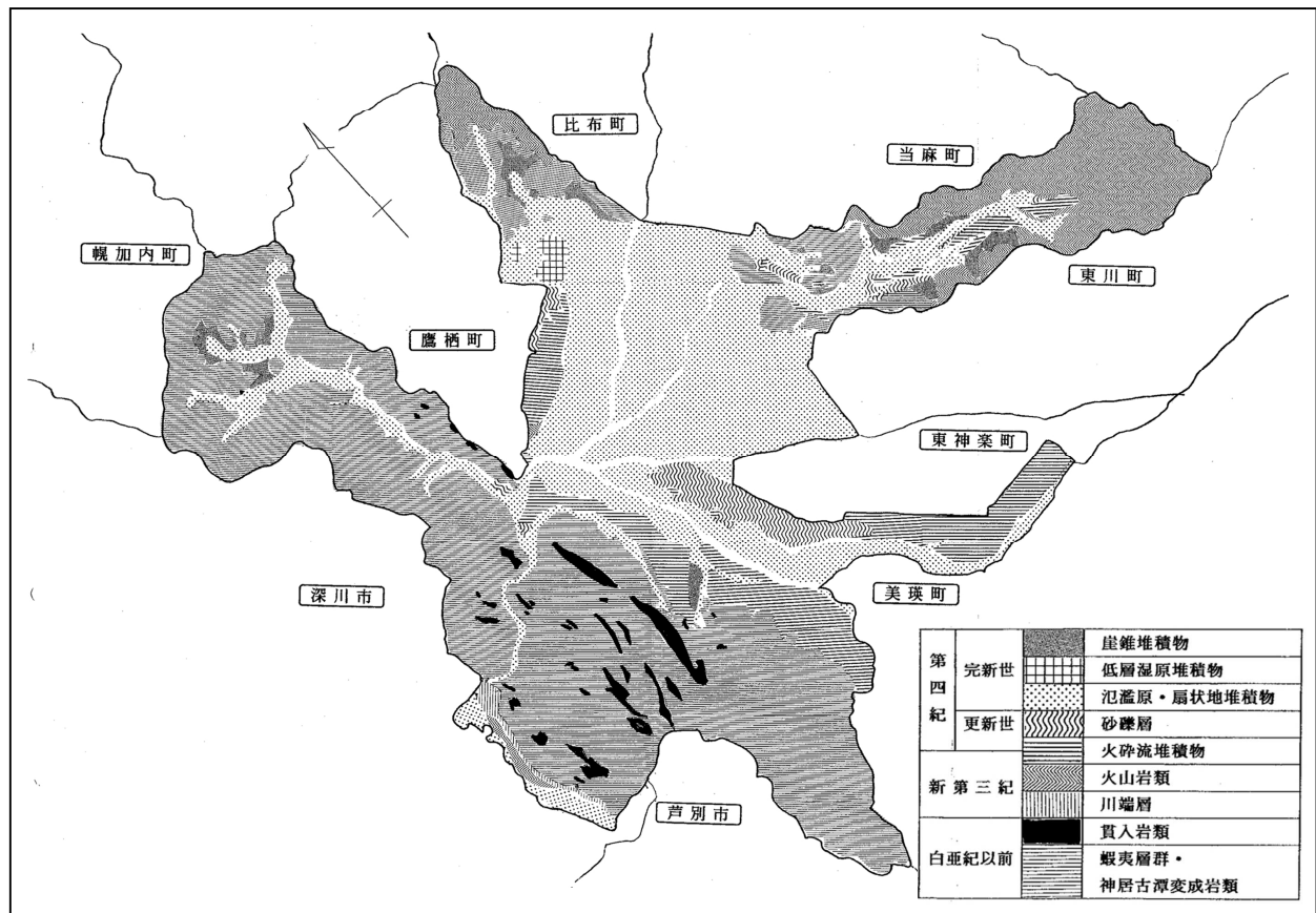
■表層地質図
