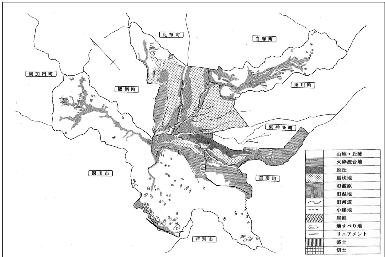
■地形分類図
