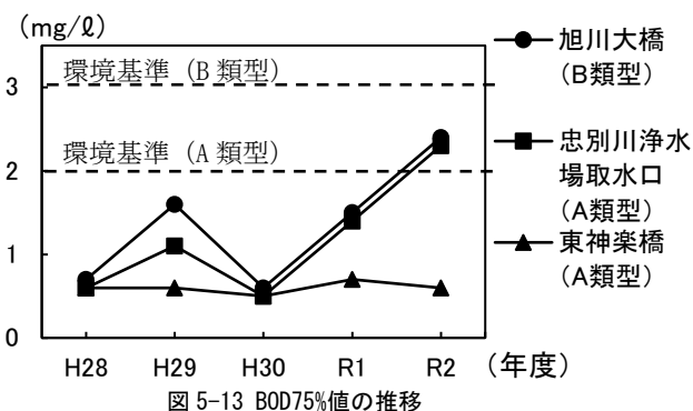
図 5-13 BOD75%値の推移
