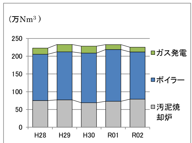
図1-3 消化ガス発生量と使用内訳の推移
