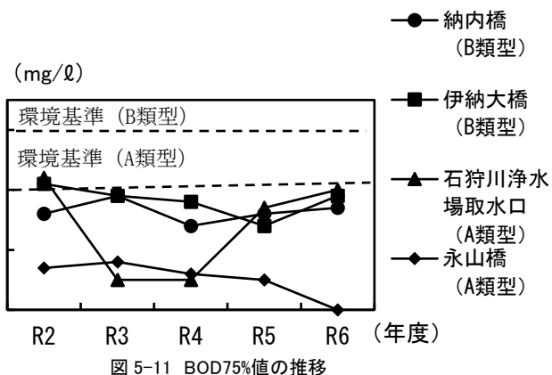
図 5-11 BOD75%値の推移
