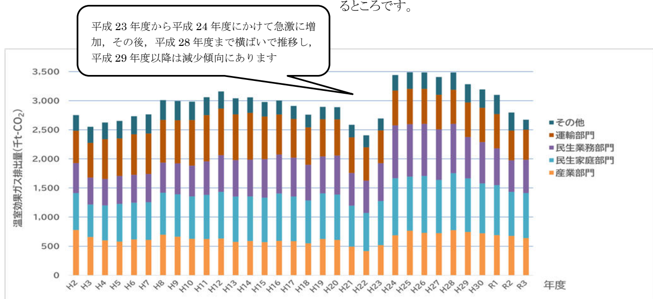
図2-1 旭川市の温室効果ガス排出量の推移
