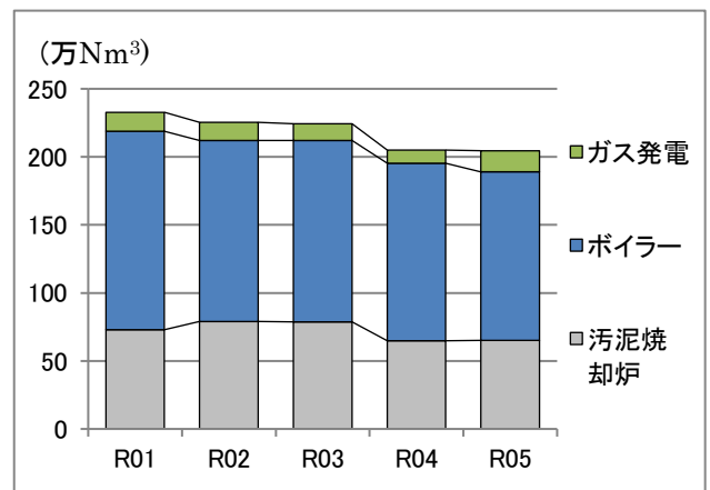
図1-3 消化ガス発生量と使用内訳の推移
