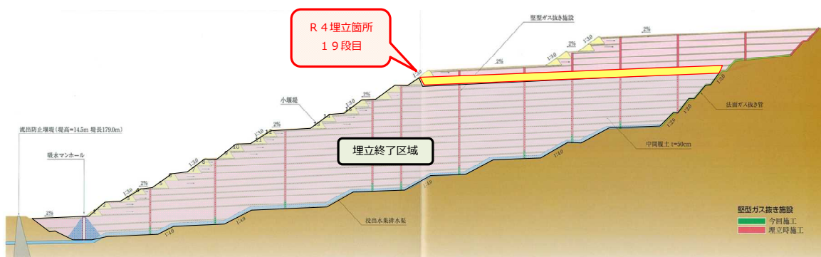
埋立地縦断面図
