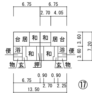
教員住宅 1階
