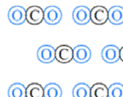
ケ 二酸化炭素 [CO 2 ]
