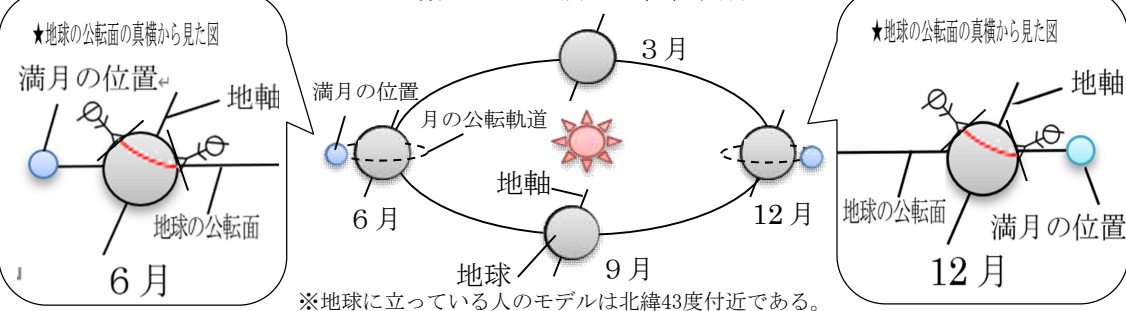
＜太陽と地球と満月の位置関係＞
