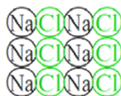
キ 食塩 [NaCl]
