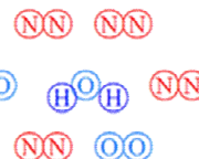
コ 空気 [N 2 , O 2 , H 2 O]
