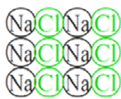
キ 食塩 [NaCl]
