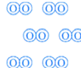
オ 酸素 [O 2 ]
