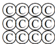
ウ 炭素 [C]
