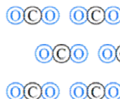
ケ 二酸化炭素 [CO 2 ]
