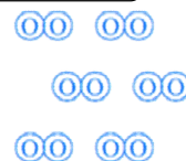
オ 酸素 [O 2 ]
