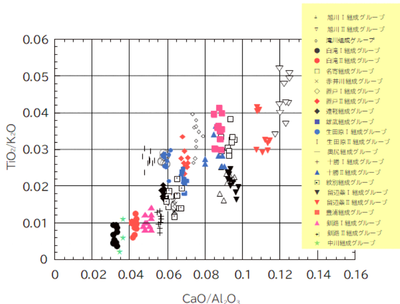
北海道内から産出した黒曜石ガラスの主成分化学組成の分析分類図
