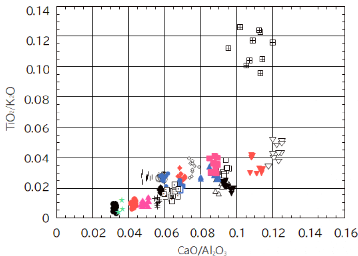
図1 北海道における \text{CaO}/\text{Al}_2\text{O}_3 - \text{TiO}_2/\text{K}_2\text{O} の関係図.
