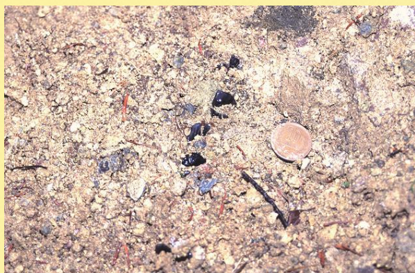
写真2 忠烈布丘陵の川西層(後期中新世)の土石流堆積物中の黒曜石。川西層中には膨大な量の黒曜石が含まれ、そこから現在でも川の中に洗い出される。
