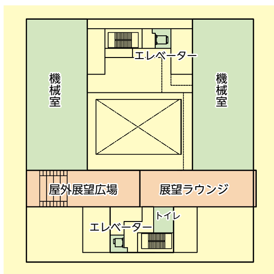
9階 平面図
