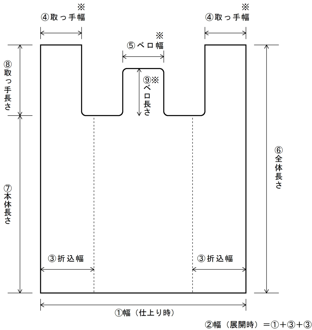
指定ごみ袋の寸法（単位：mm）
