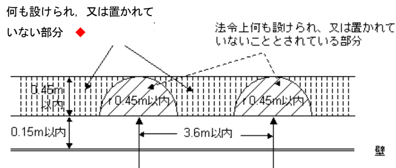
〔側壁型ヘッドの場合：平面〕
