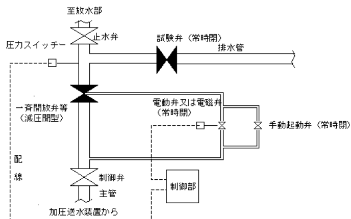
図6 〔加圧方式の一斉開放弁等の廻りの配管図例〕
