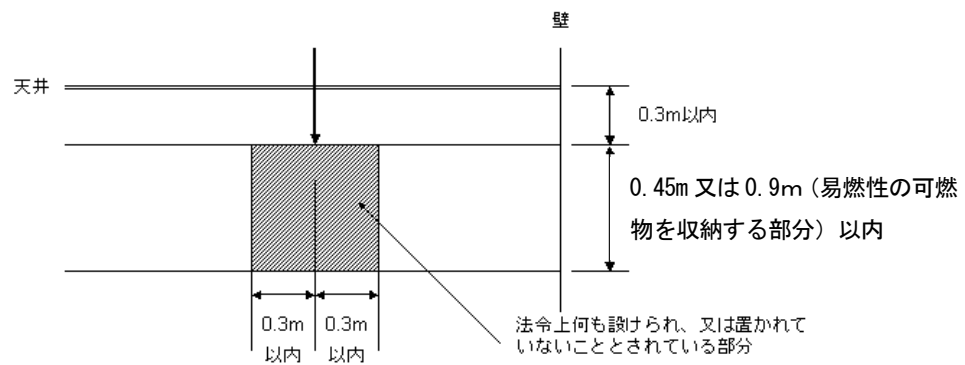
〔標準型ヘッド（小区画型ヘッドを除く。）：断面〕
