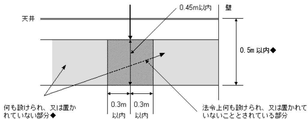
〔小区画型ヘッドの場合：断面〕
