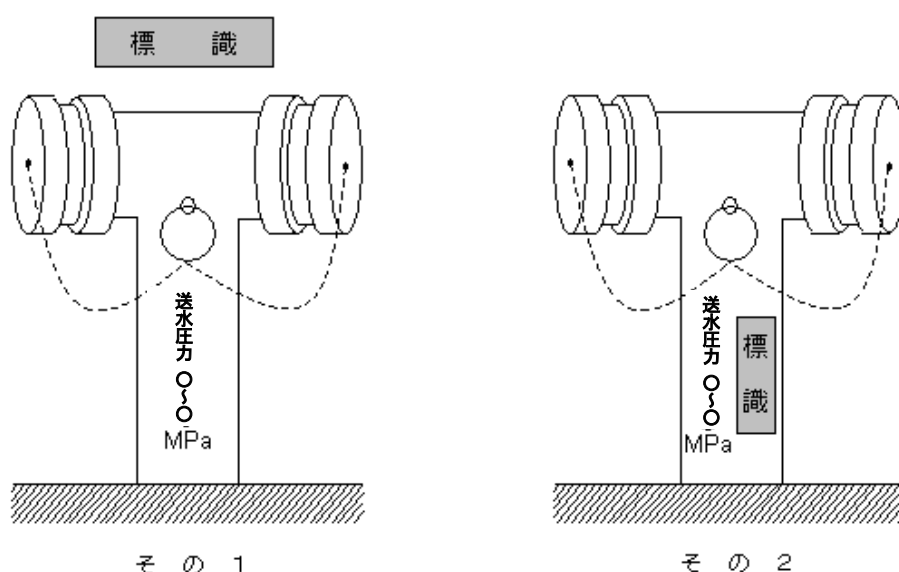
〔スタンド型の例〕 第3-6図
