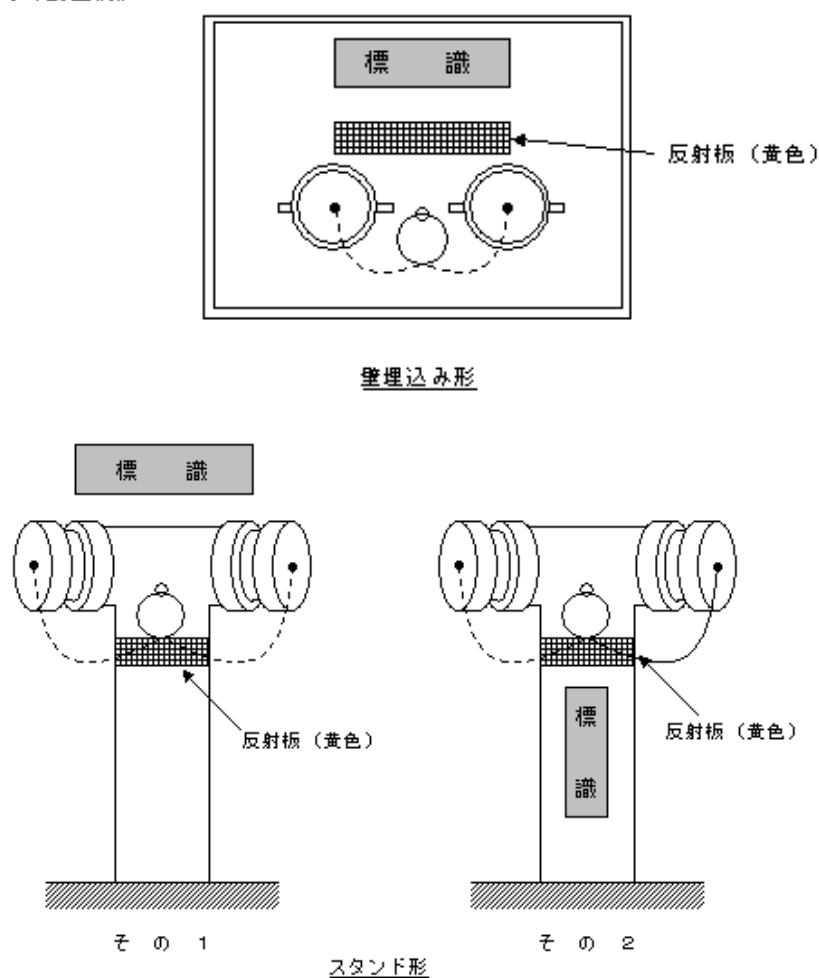
第 21-5 図 連結送水管の送水口の標識等
