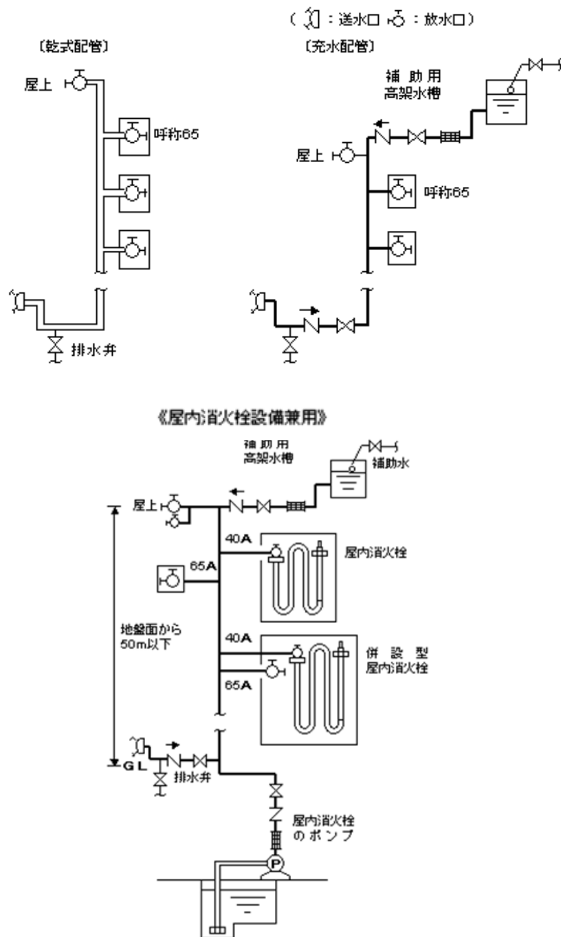
第 21-1 図 連結送水管の配管図例
