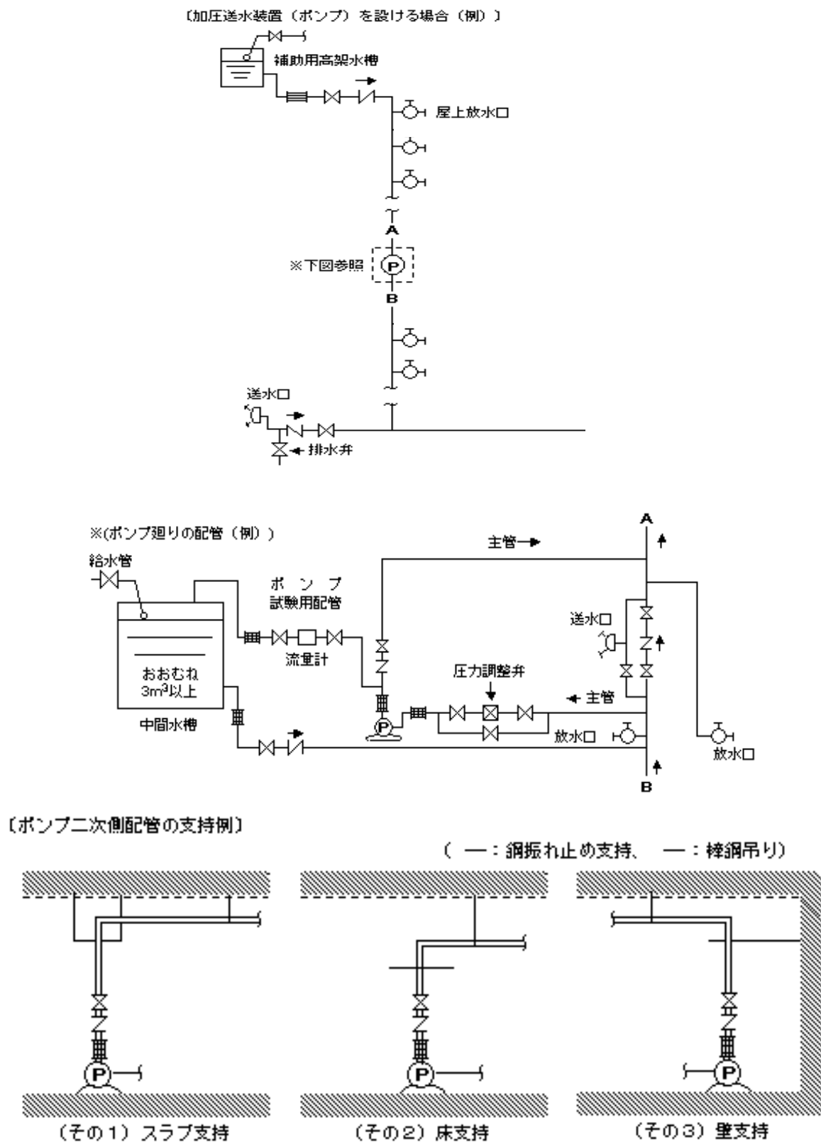
第 21-3 図 プースターポンプを設置する場合の配管例
