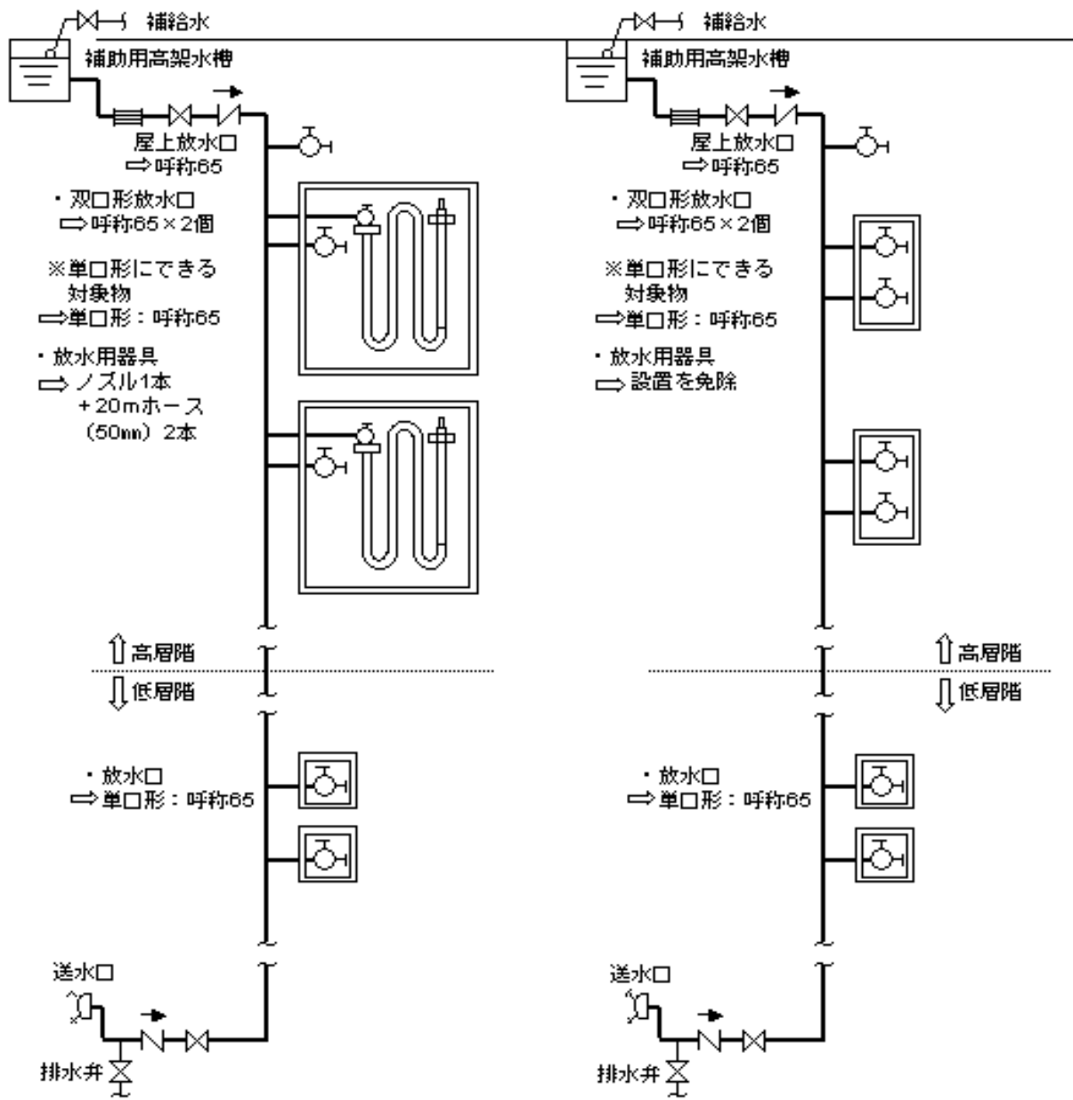
第 21- 2 図 連結送水管の配管例〔高層建築物等に設ける場合〕
