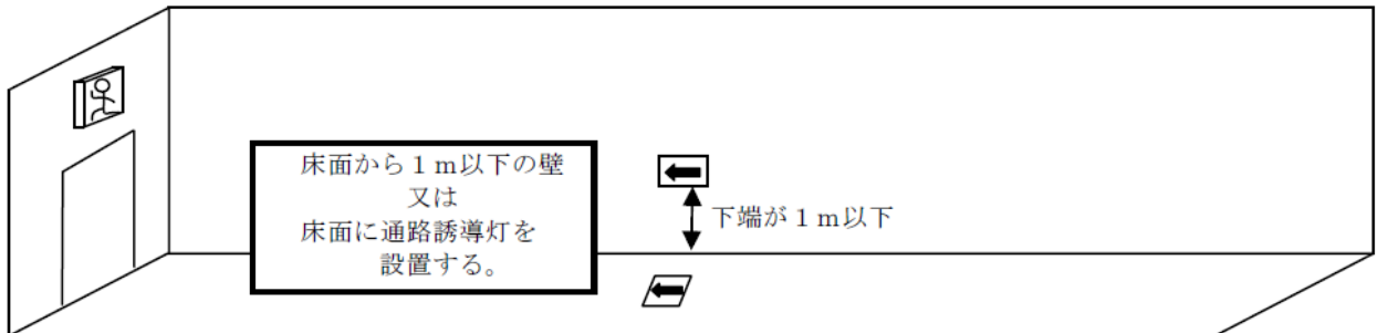
図 1 省令第28条の3第4項第3号の2により誘導灯を設置した場合
