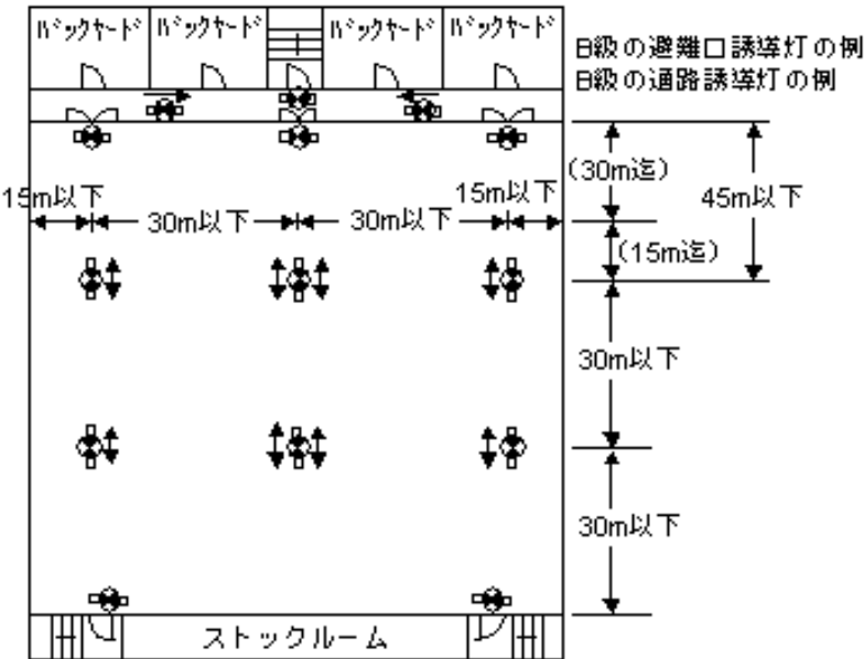
第 17－4 図 居室の各部分から誘導灯を見とおしできる場合の設置例
