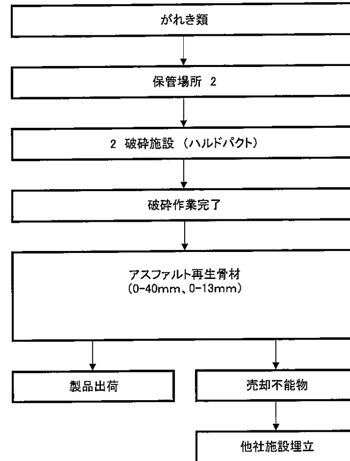
がれき類(アスファルト)破碎施設フロー図
