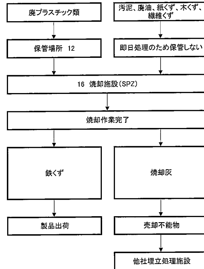
焼却施設フロー図
