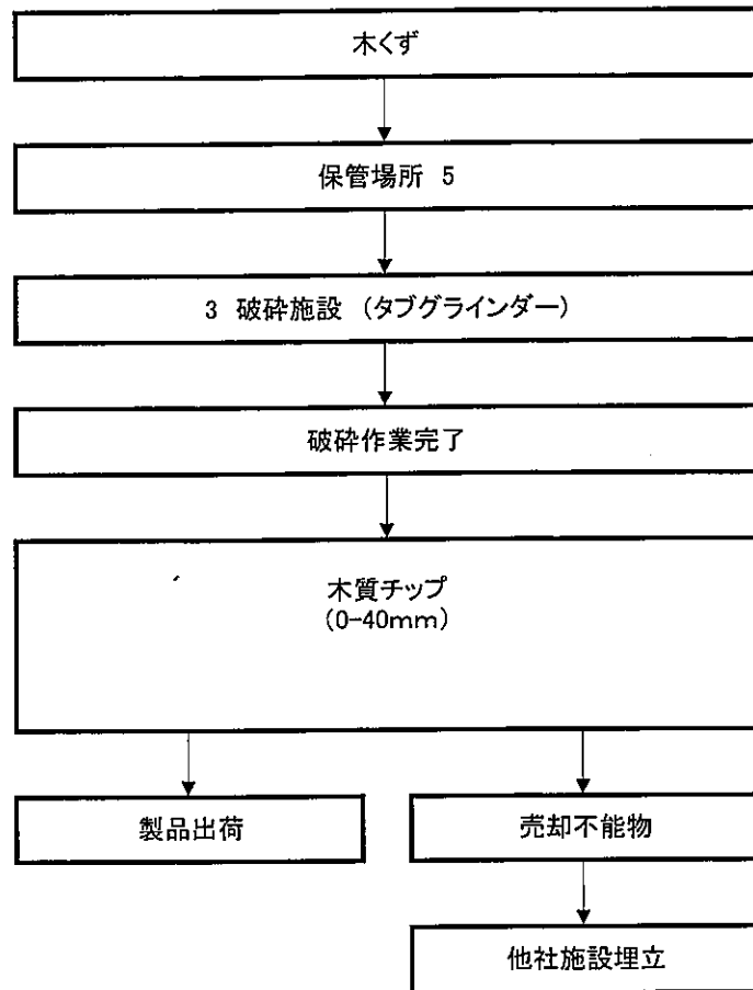
木くず破碎施設フロー図
