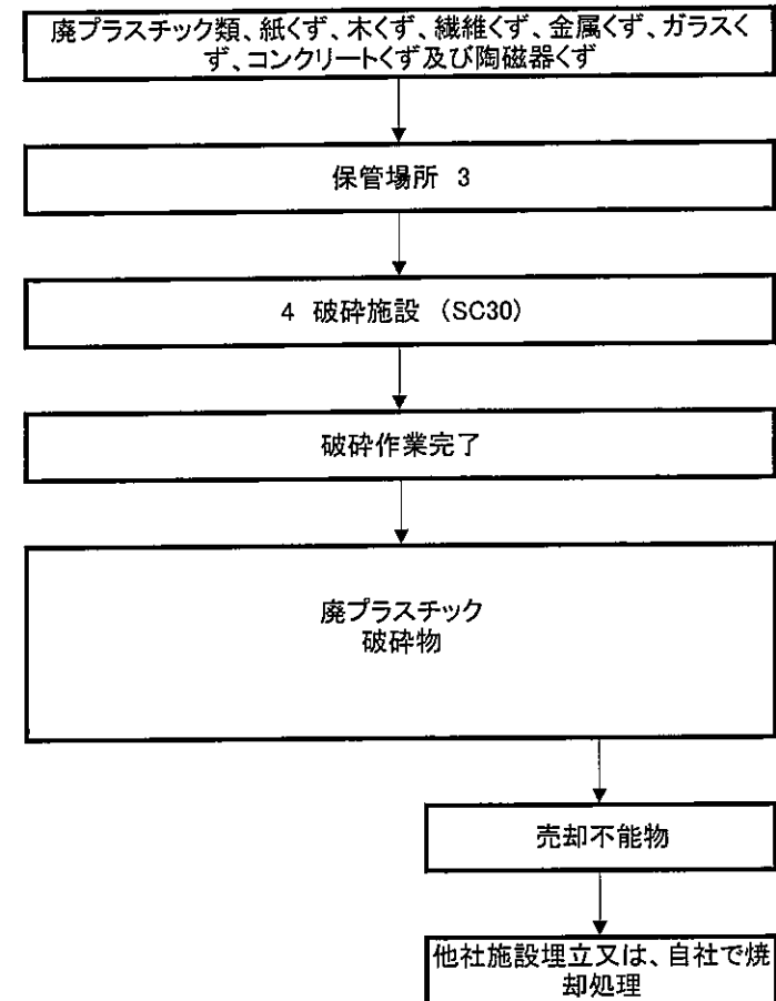
廃プラスチック類、紙くず、木くず、繊維くず、金属くず、ガラスくず、コンクリートくず及び陶磁器くず破碎施設フロー図
