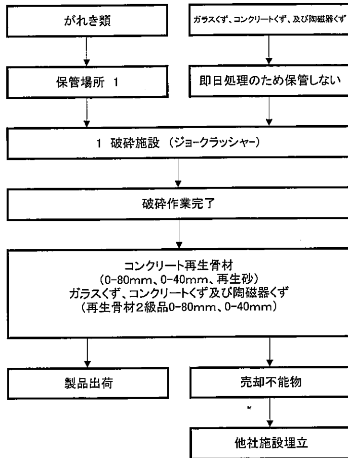
がれき類(コンクリート)破碎施設フロー図
