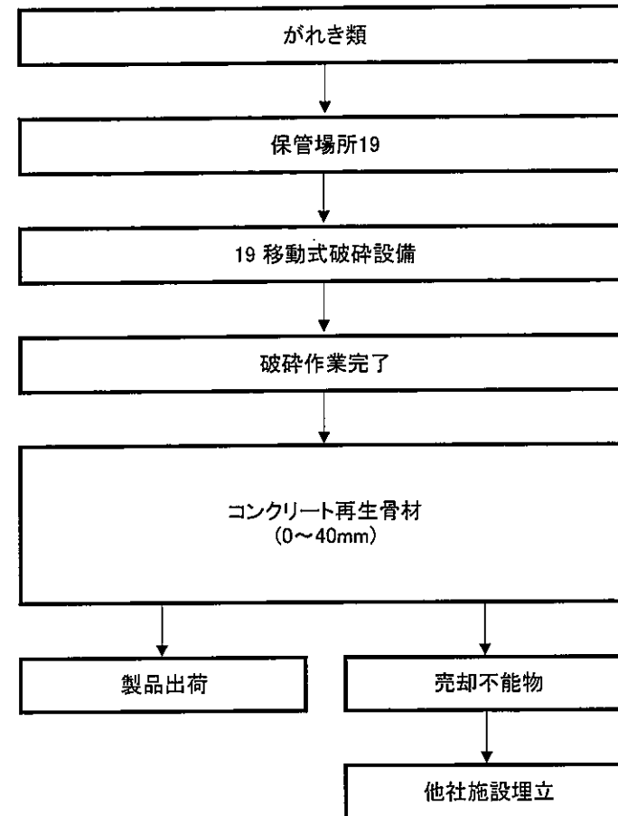
がれき類(アスファルト)破碎施設フロー図
