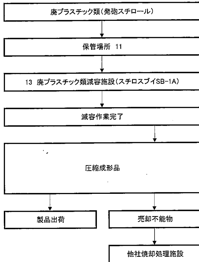
廃プラスチック類減容施設フロー図
