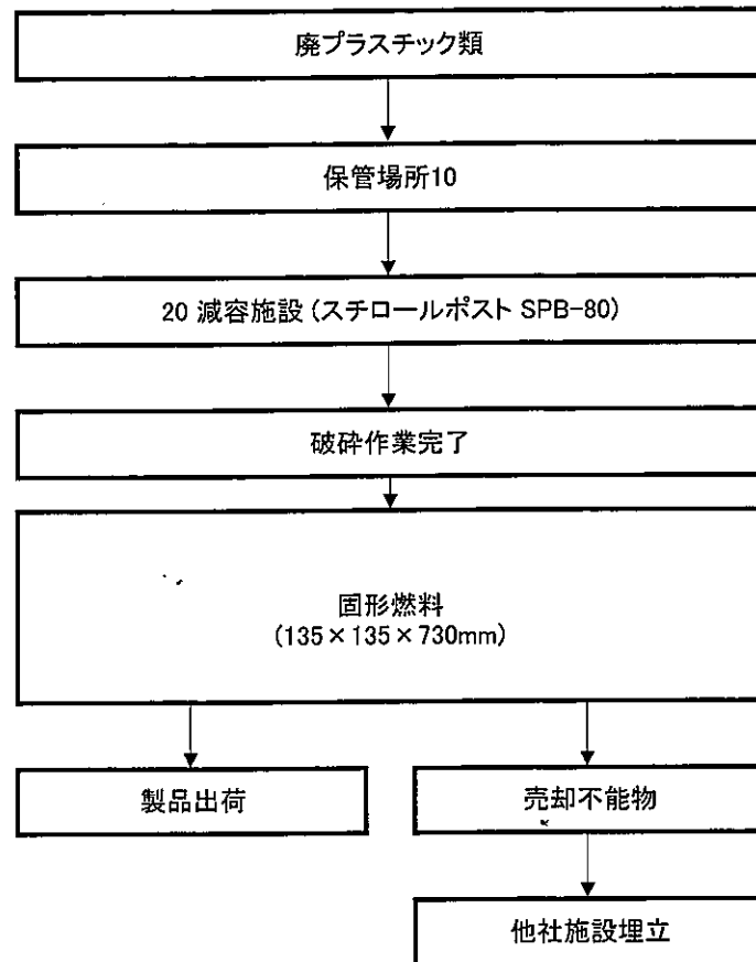
廃プラスチック類(発砲・スタイロ)減容施設フロー図
