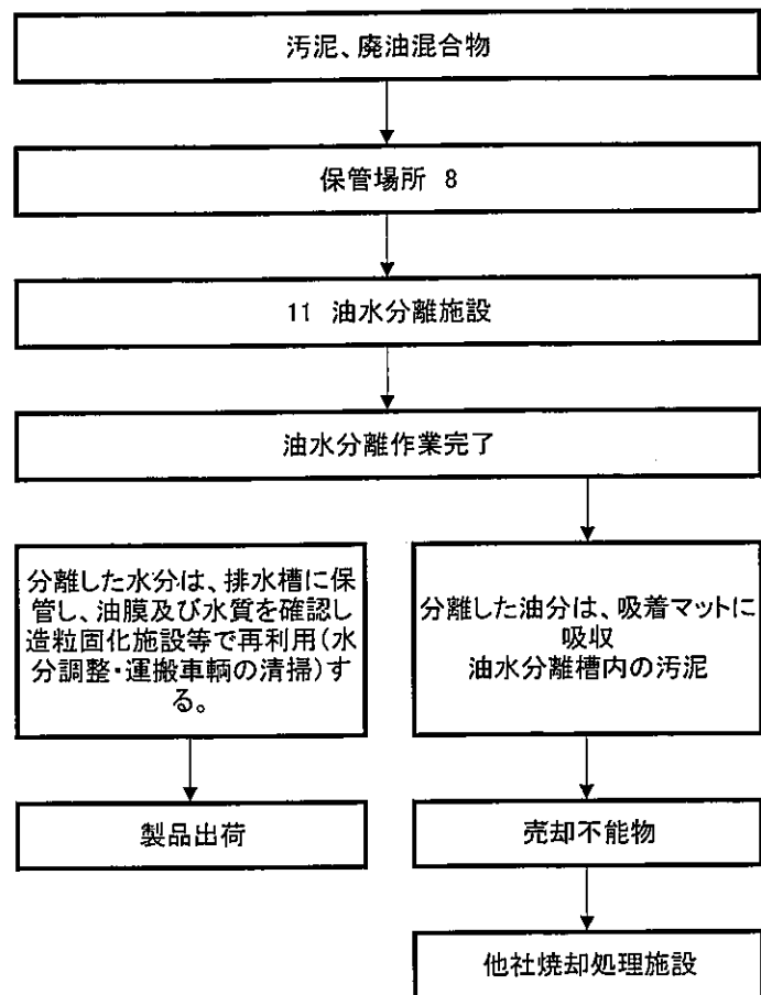
汚泥、廃油油水分離施設フロー図
