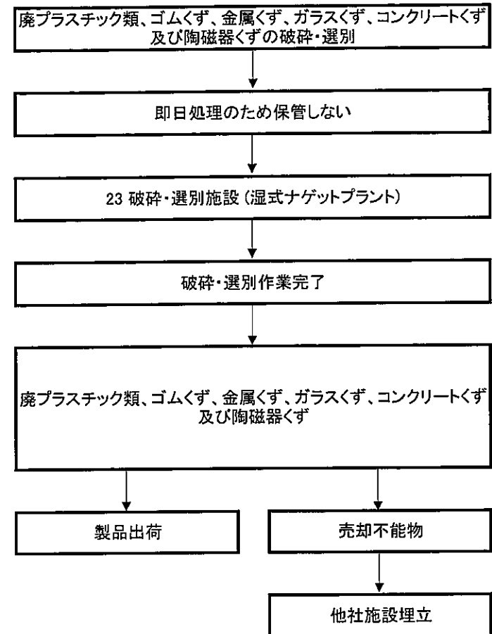
廃プラスチック類、ゴムくず、金属くず、ガラスくず、コンクリートくず及び陶磁器くずの破砕・選別施設フロー図
