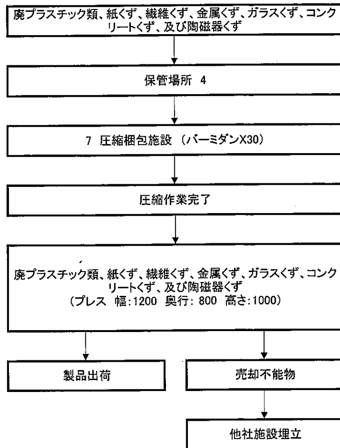
圧縮梱包施設フロー図
