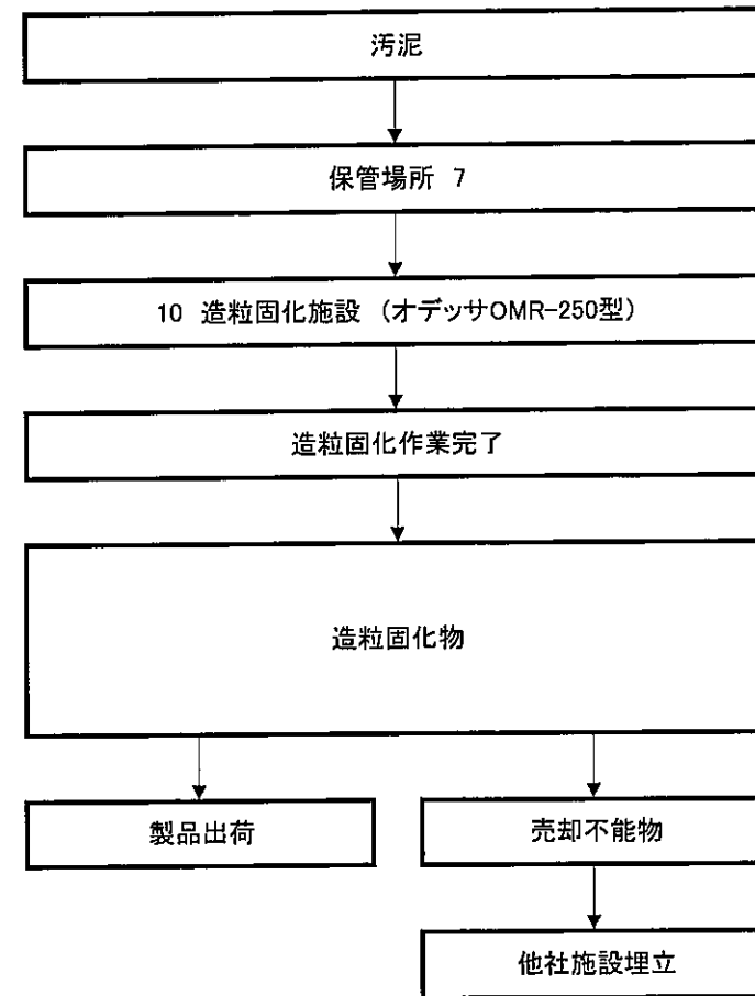
汚泥造粒固化施設フロー図
