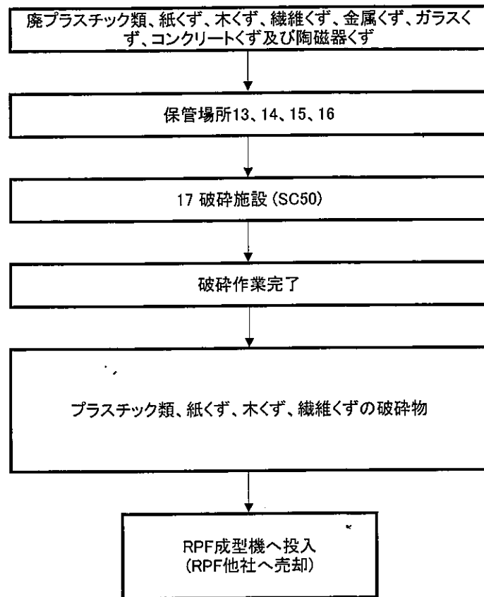
廃プラスチック類、紙くず、木くず、繊維くず、金属くず、ガラスくず、コンクリートくず及び陶磁器くず破碎施設フロー図
