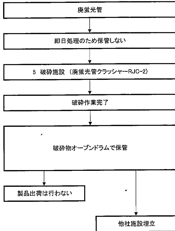
廃蛍光管破碎施設フロー図
