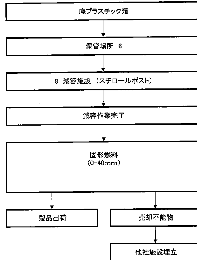
廃プラスチック類(発砲・スタイロ)減容施設フロー図
