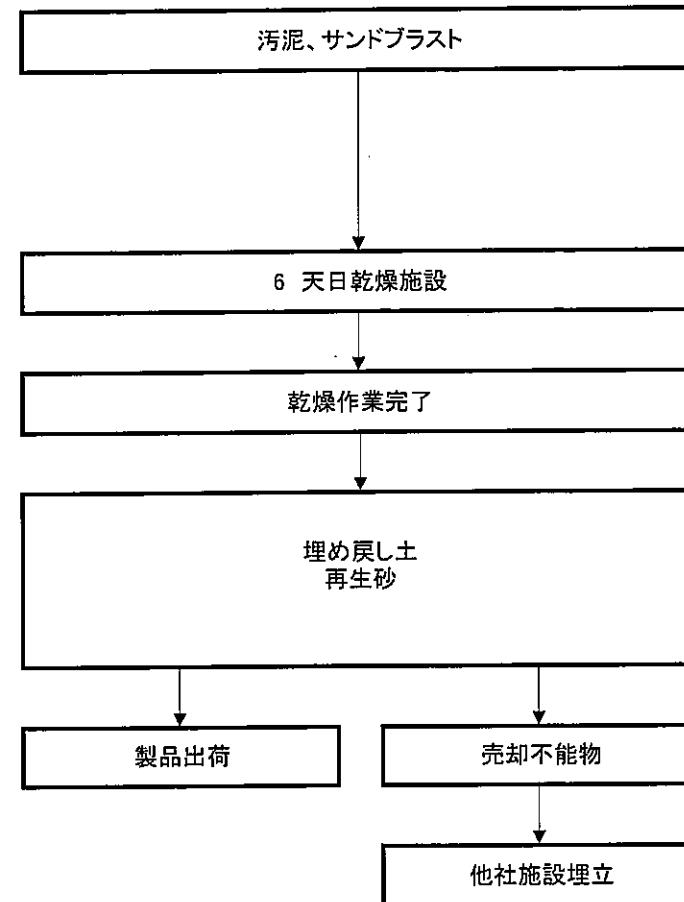
汚泥の天日乾燥施設フロー図
