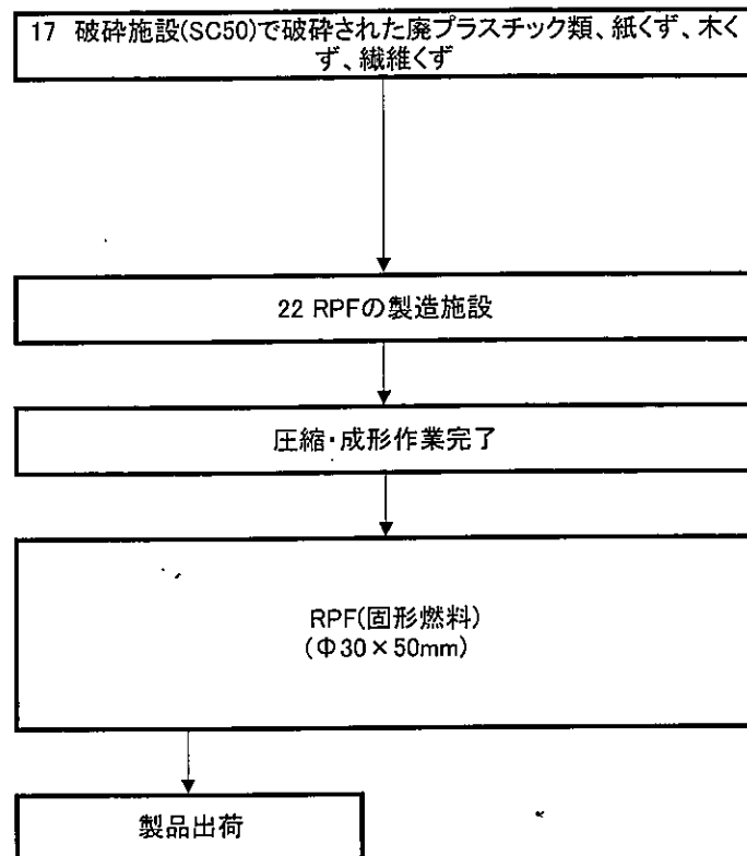
廃プラスチック類、紙くず、木くず、繊維くずの圧縮・施設フロー図
