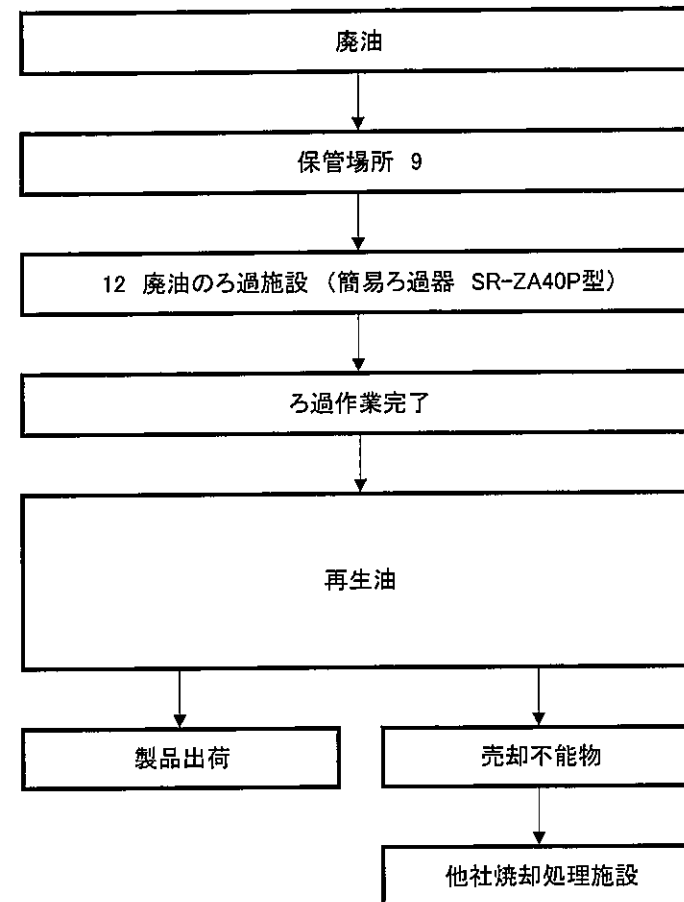
廃油のろ過施設フロー図
