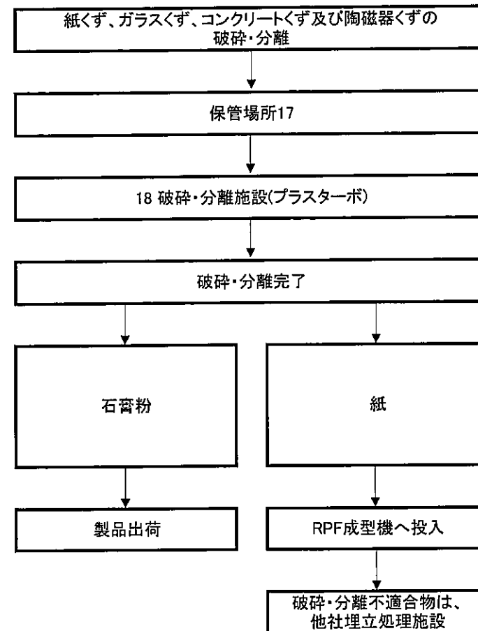
紙くず、ガラスくず、コンクリートくず及び陶磁器くずの破碎・分離フロー図
