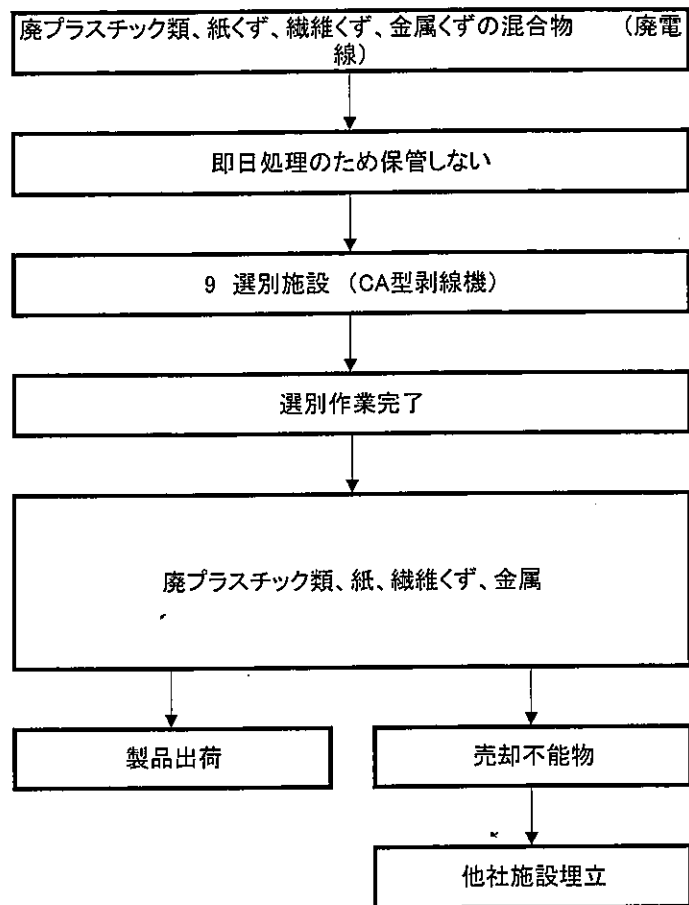
選別施設フロー図
