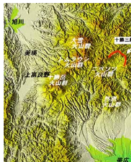
図表 1-3 旭川市周辺の火山群
