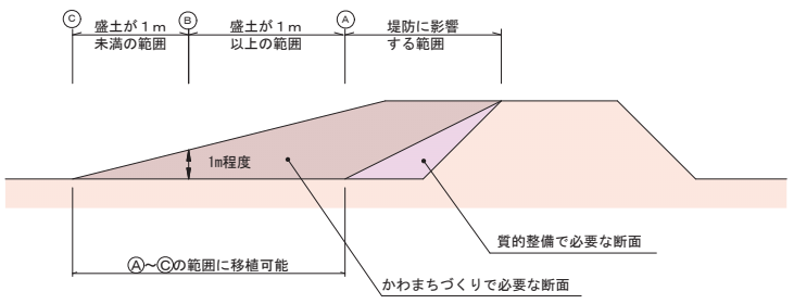
築堤断面図
