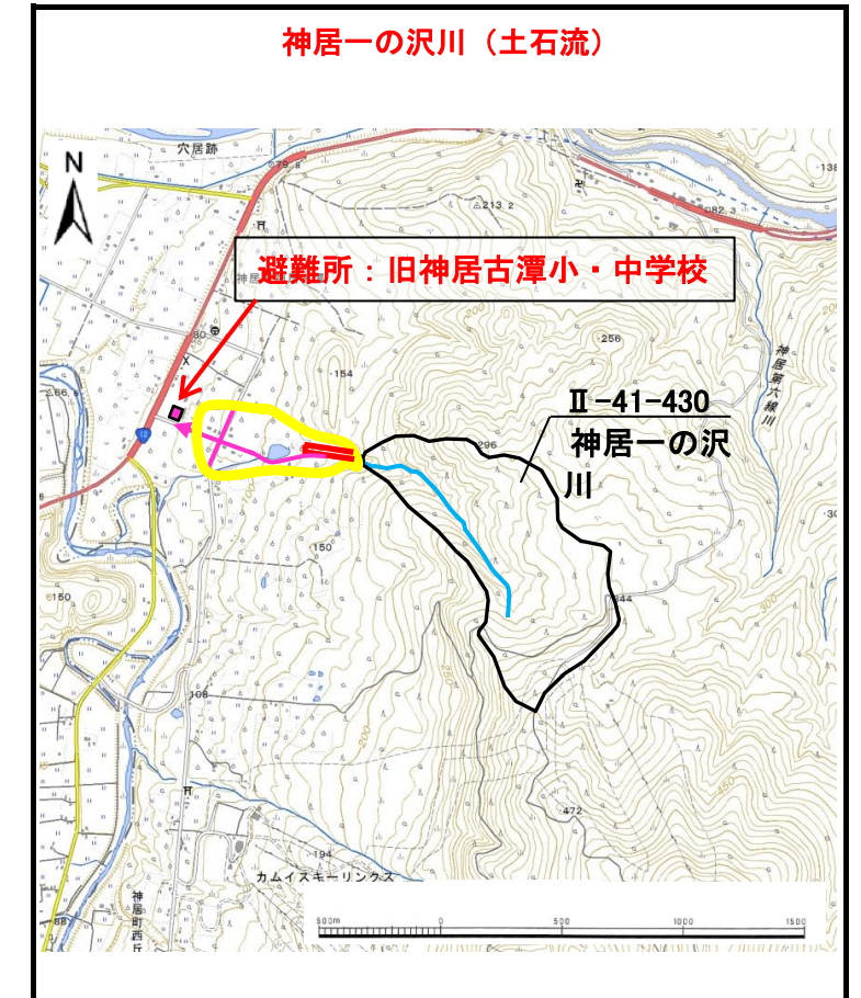
位置図
