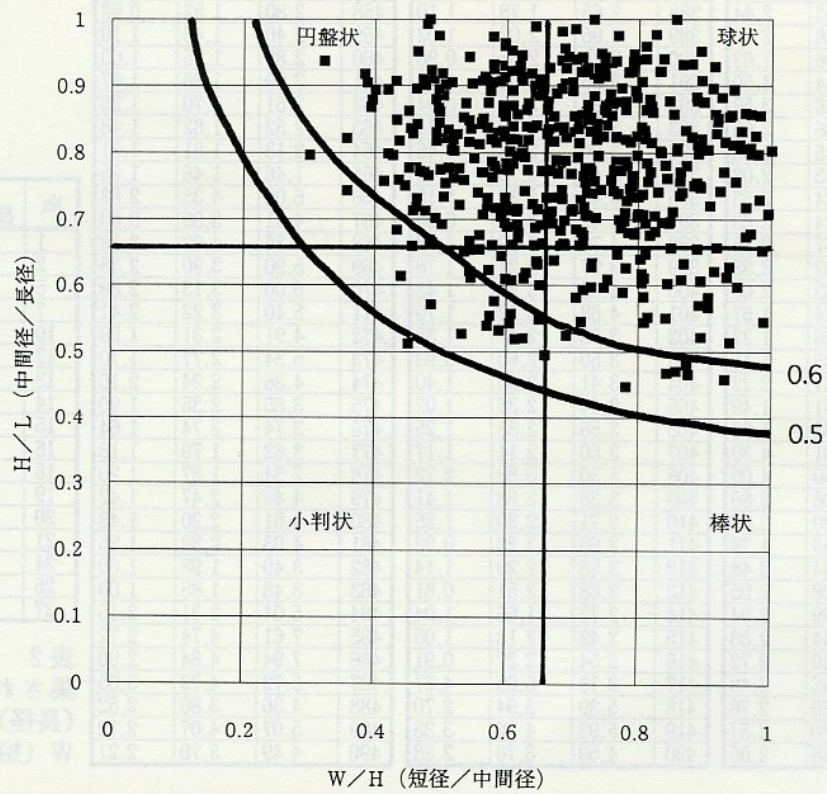
図4 近文台北西部より産出した黒曜石礫の形状分類 (Zingg,1935) と球形度曲線 (Krumbein,1941)
