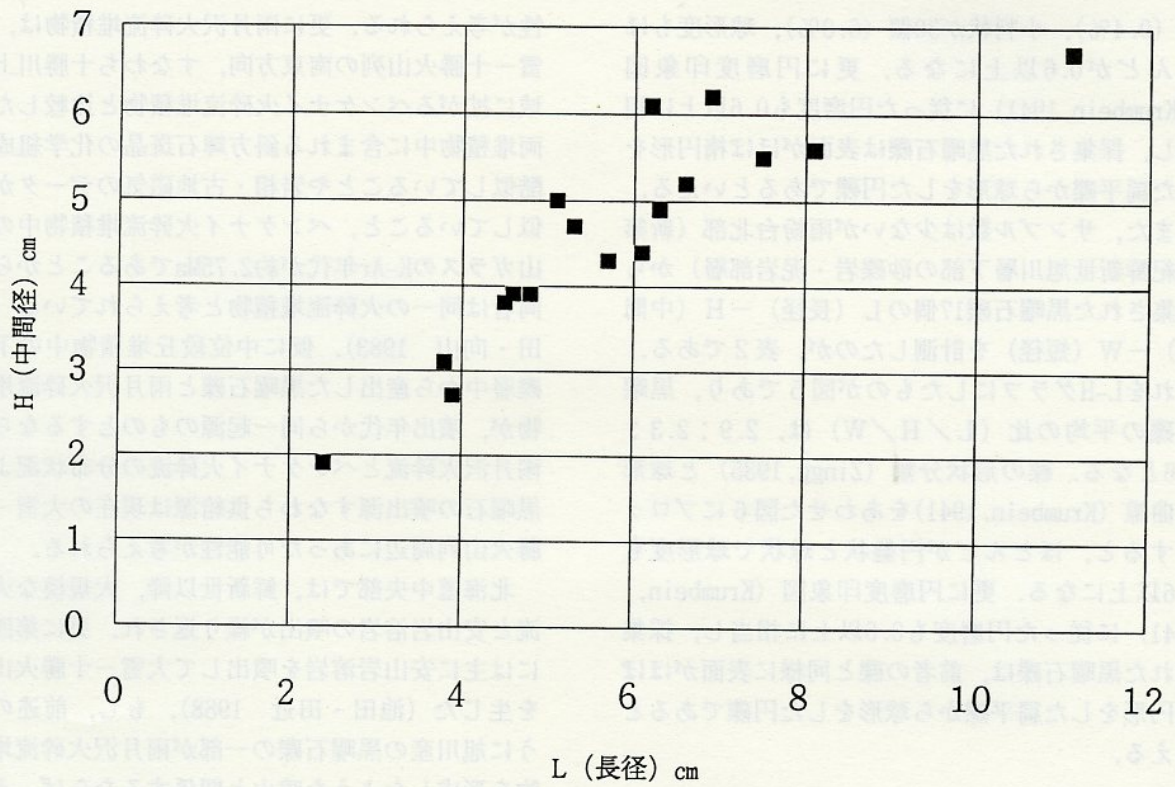
図5 雨舂台北部から採集された黒曜石のL-Hグラフ
