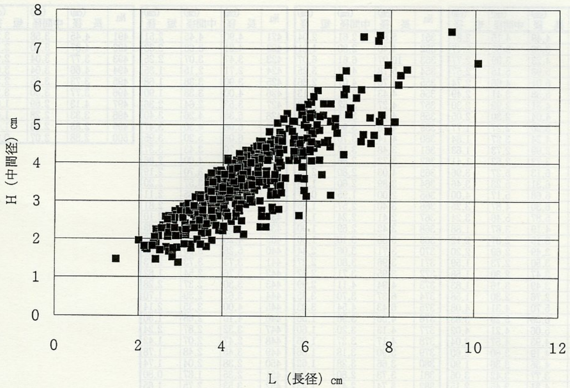
図3 近文台北西部から採集された黒曜石のL-Hグラフ
