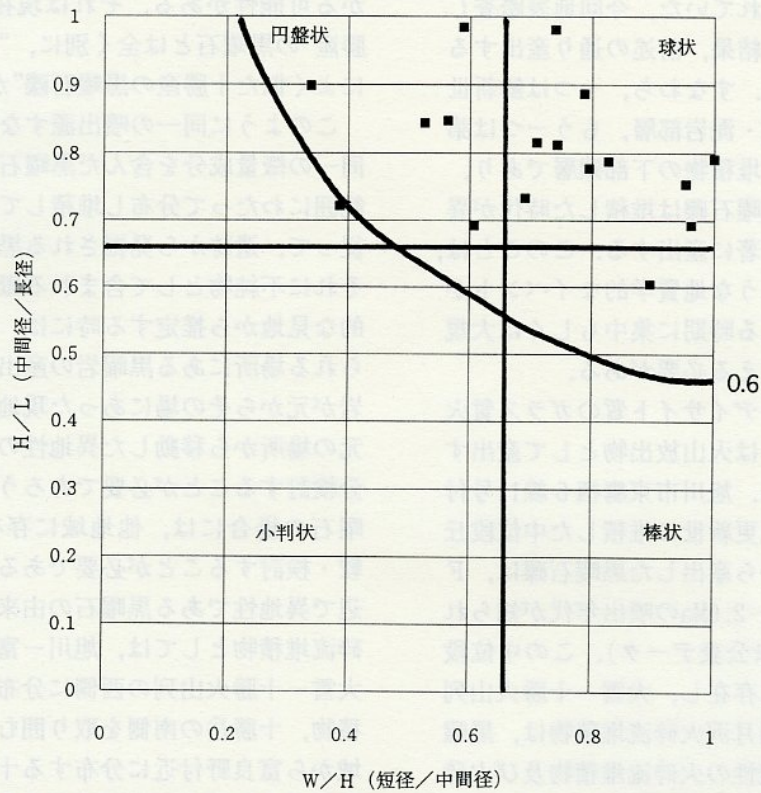
図6 雨舂台北部より産出した黒曜石礫の形状分類 (Zingg, 1935) と球形度曲線 (Krumbein, 1941)
