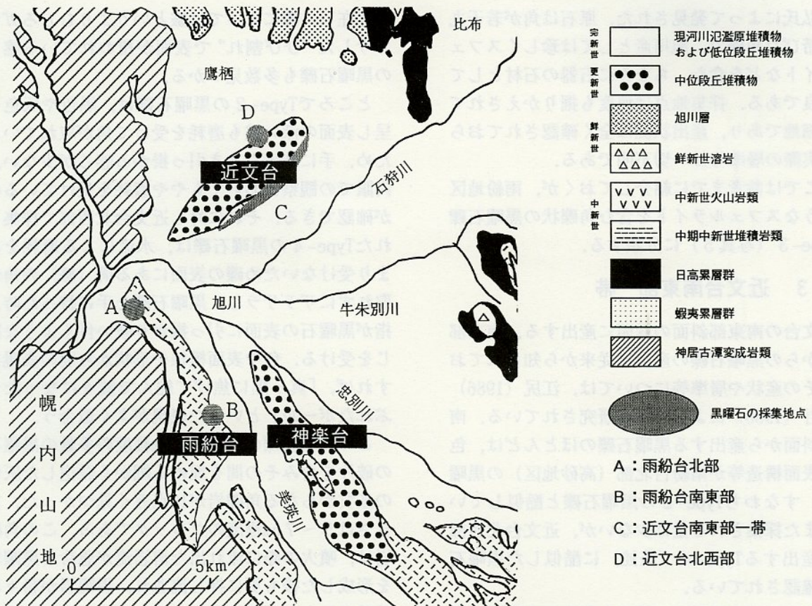
図2 台地から産出する黒曜石礫の採集地点
