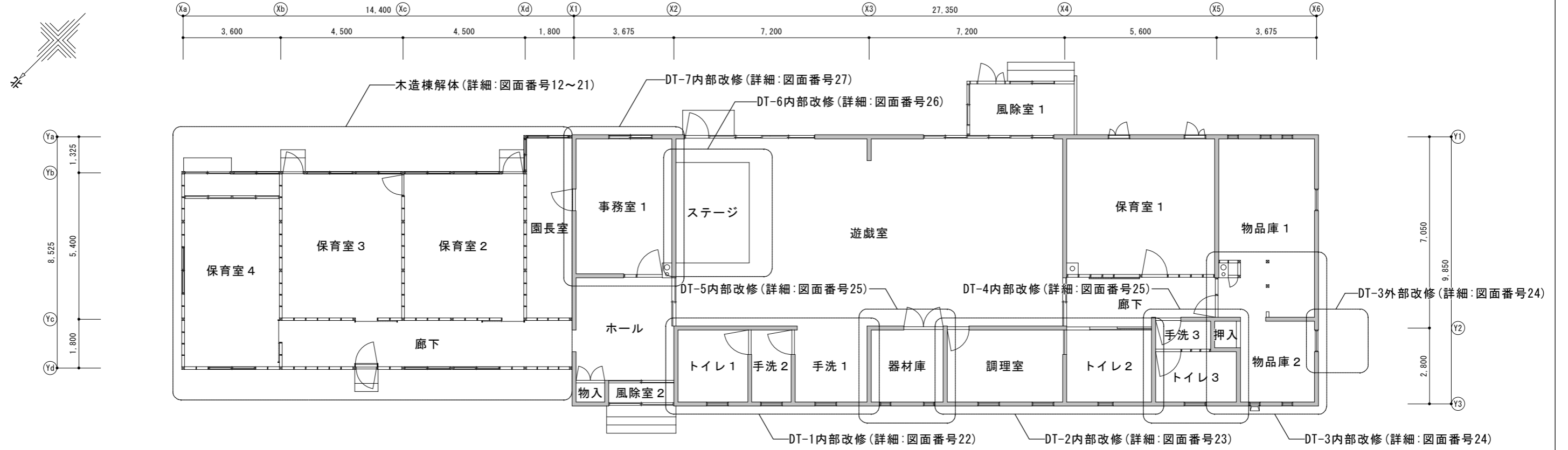
(改修前) 平面図
