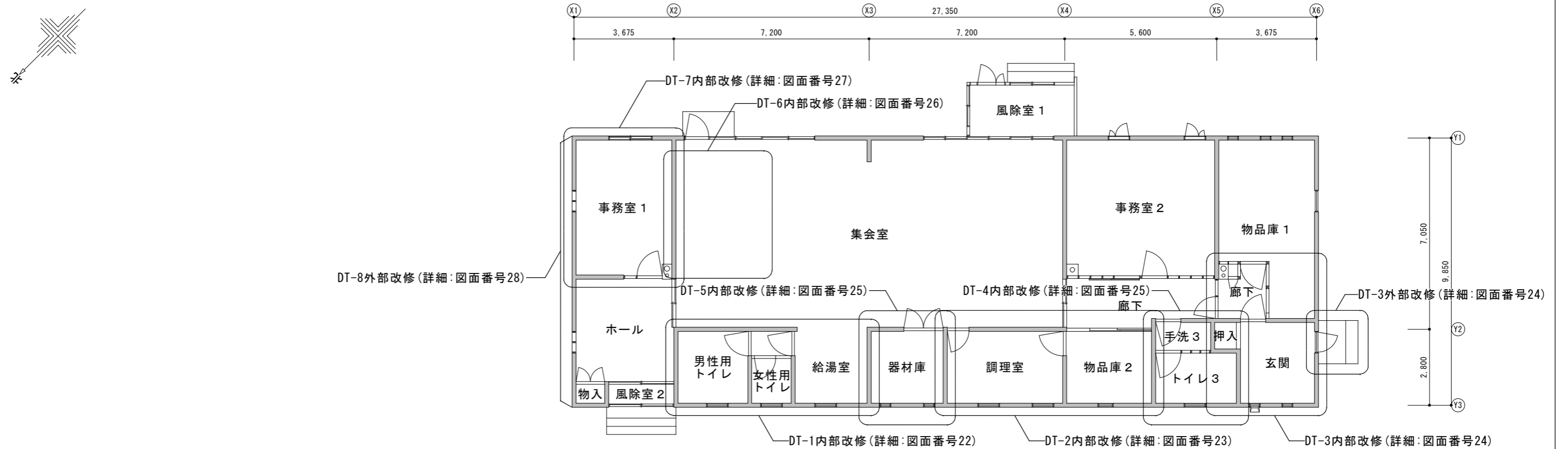
(改修後) 平面図
